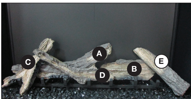
BÛCHE C : VUE DÉTAILLÉE DE L'INSTALLATION
