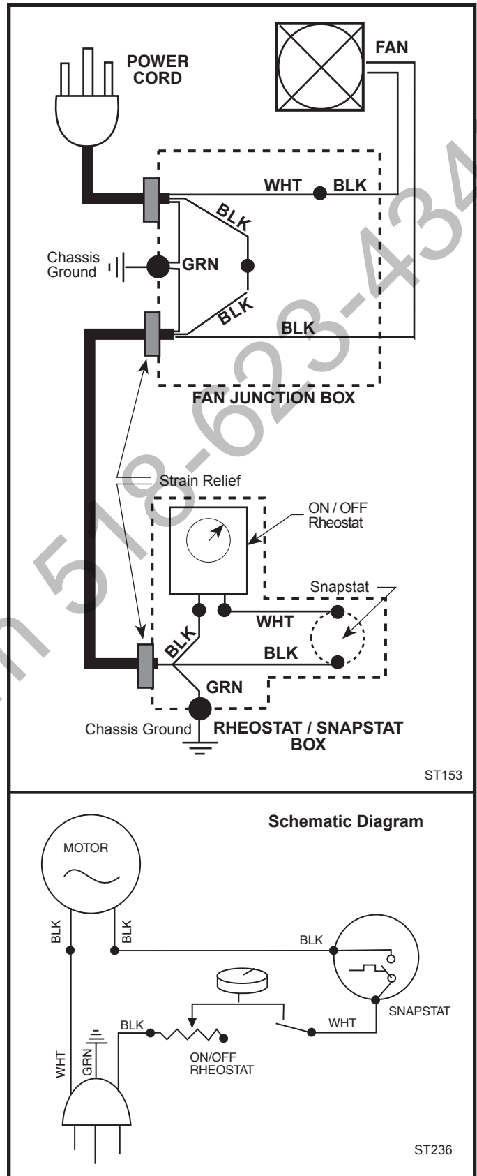
Fig. 63 Fan circuit.
