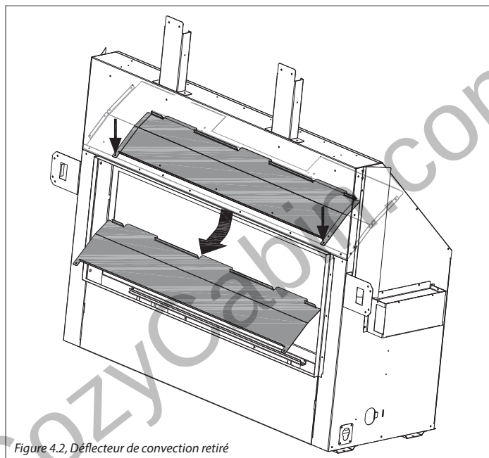
Figure 4.2, Déflecteur de convection retiré
