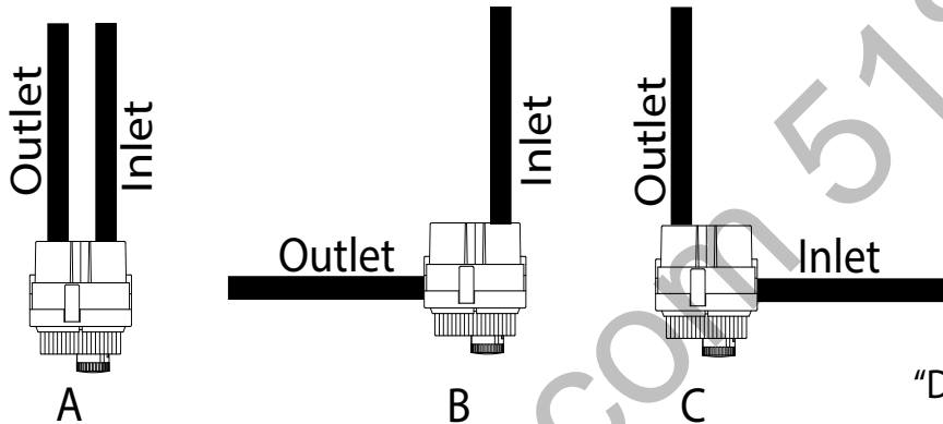
Fig. 3 Plumbing options
