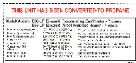
E63/E65 Conversion Decal: 908-175
