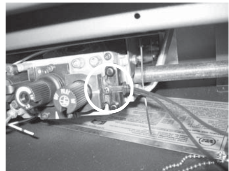
Piezo Ignitor
