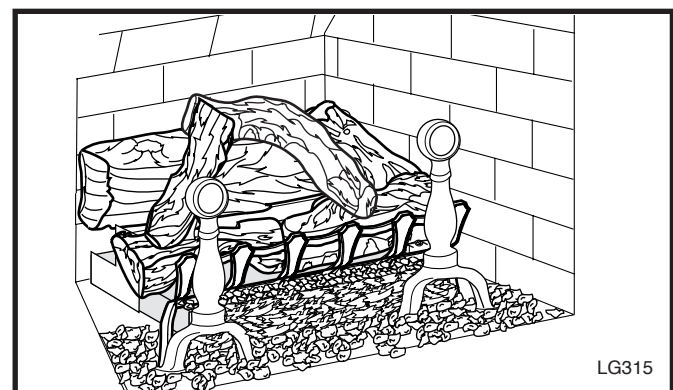
Fig. 48 DVT38 logset.
